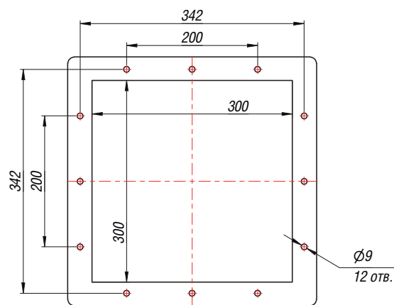
Выходной фланец
