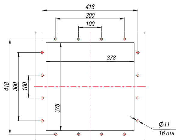
Выходной фланец
