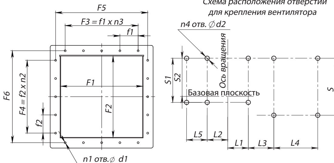
Вид E
