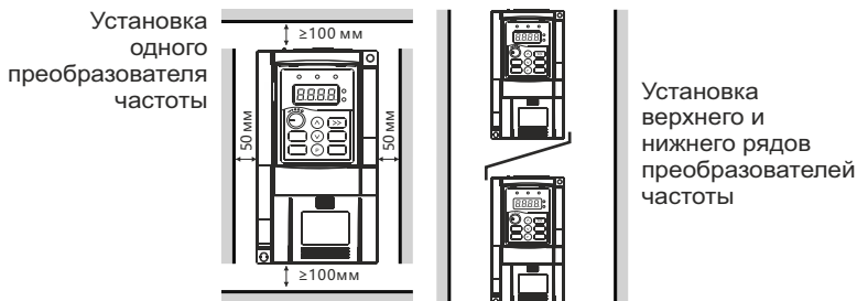
Рисунок 3-1. Схема установки
